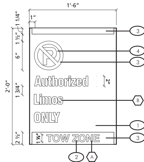
SIGN FACE LAYOUT Scale: 3/4" = 1'-0"
