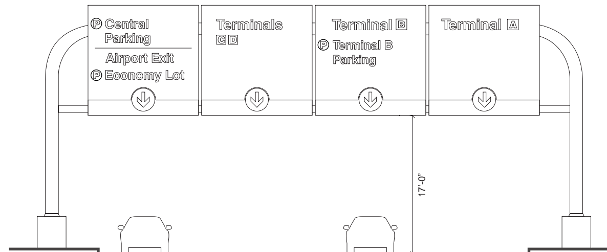
ELEVATION Scale: N.T.S.
