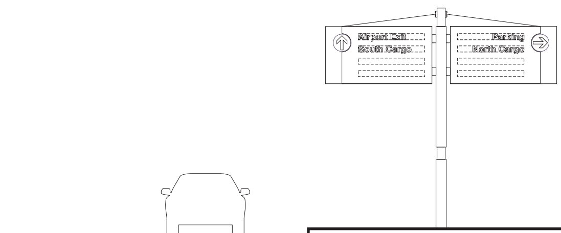
ELEVATION Scale: 1/8" = 1'-0"
